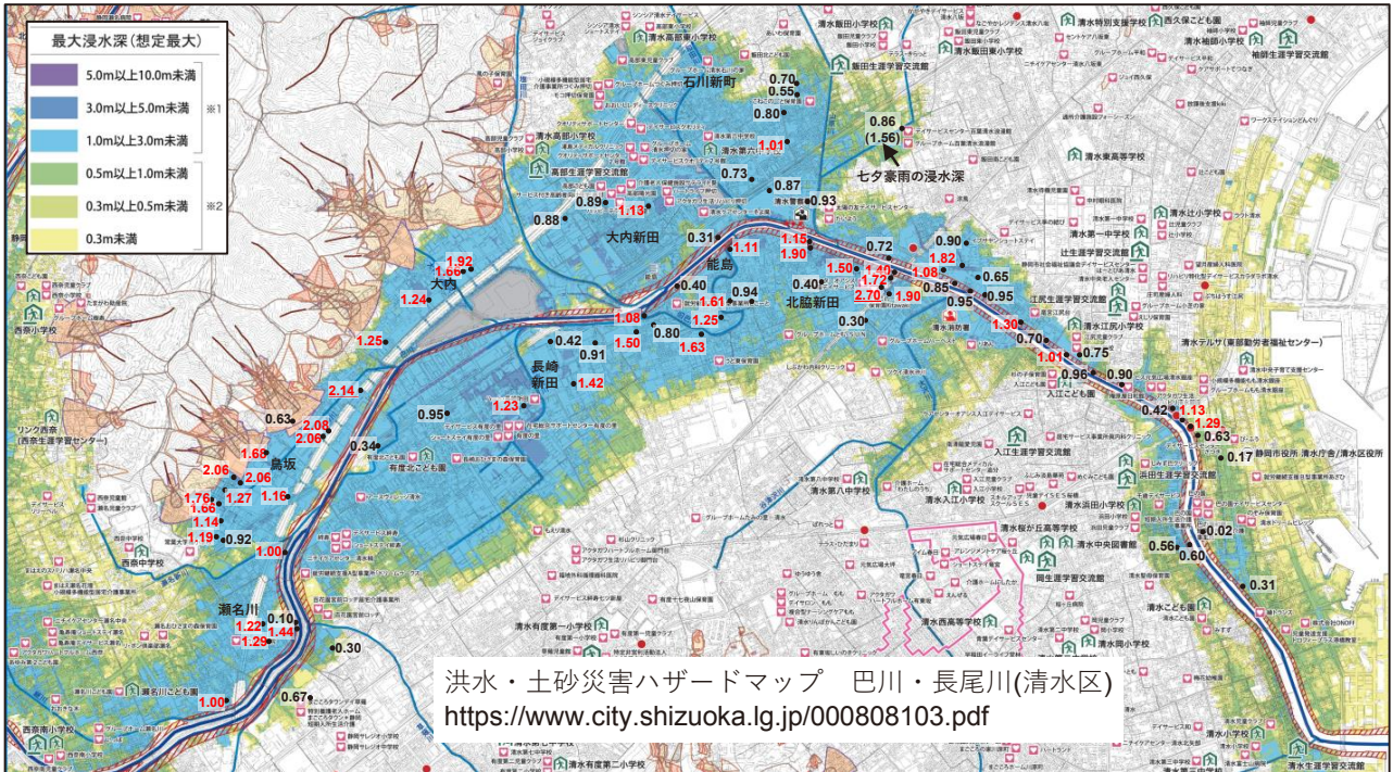
図9 調査地域の調査地点(青丸)の浸水深(m)。地図は洪水・土砂災害ハザードマップ(静岡市, 2022)。赤字は1m以上の浸水深の値である。地点22(2.14m)と55(2.70m)はアンダーパスで周辺より低くなっているので、それらの浸水深には下線を付した。
