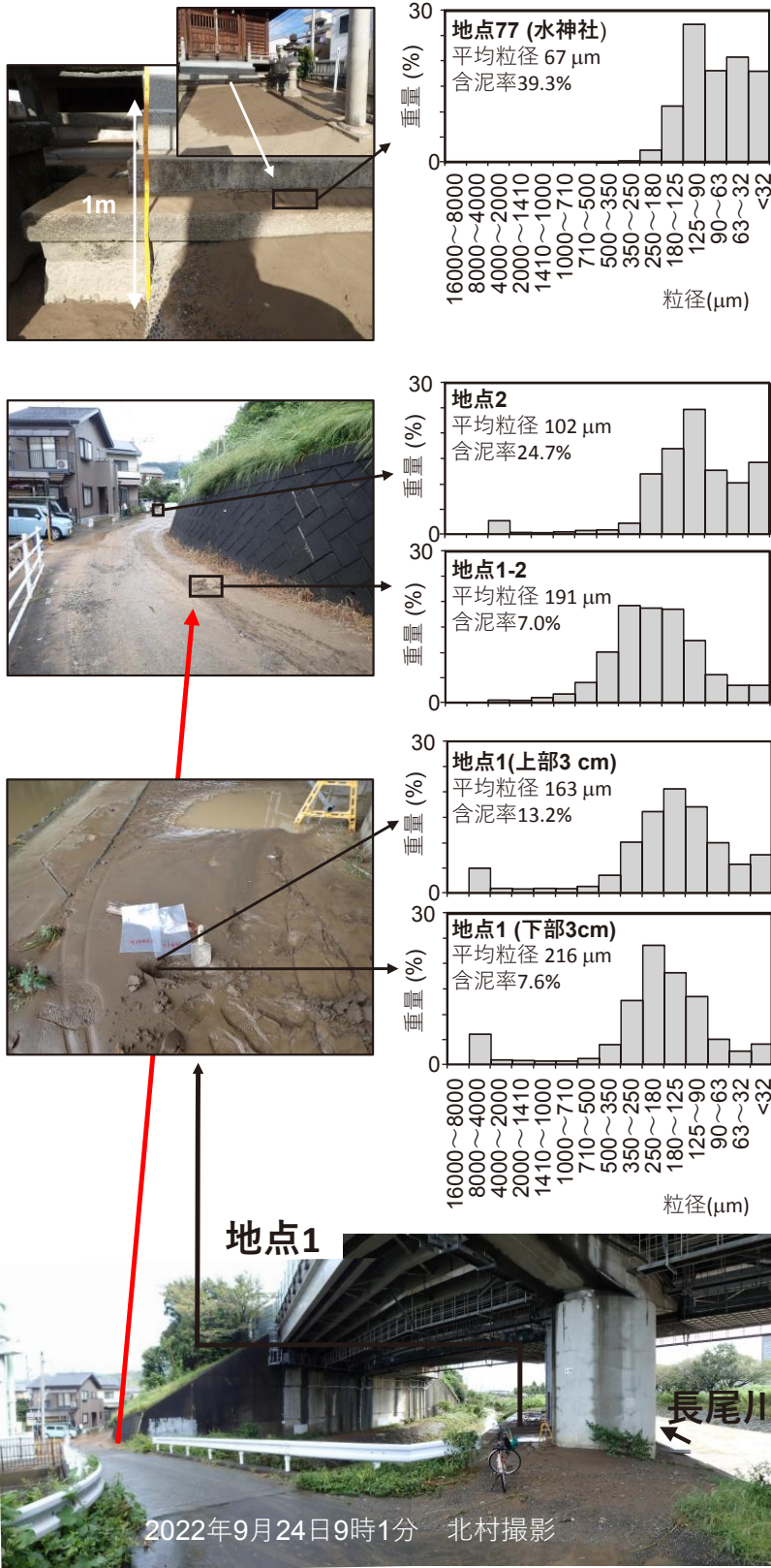
図13 洪水堆積物の粒度組成.
